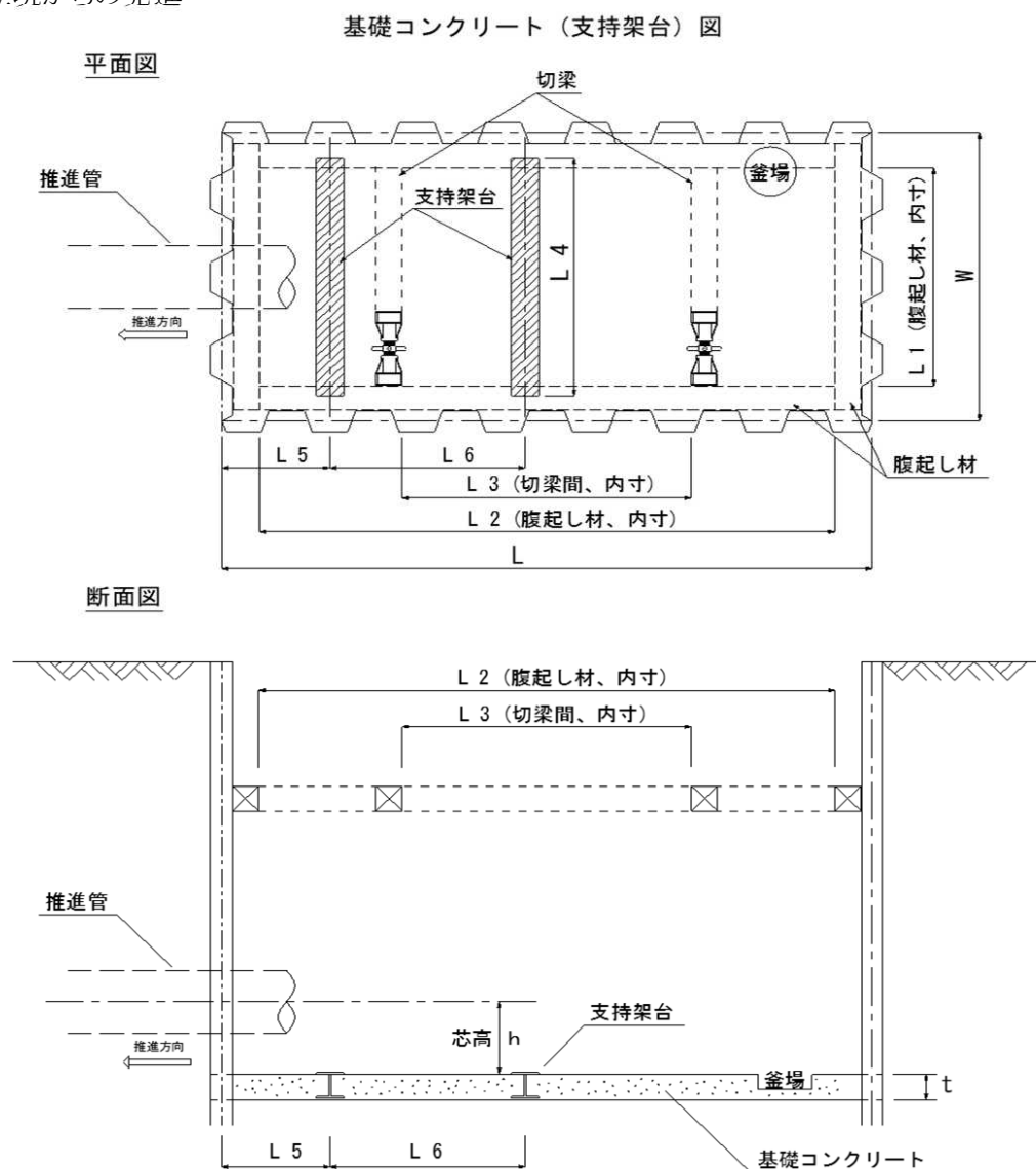
図-17 矩形立坑
