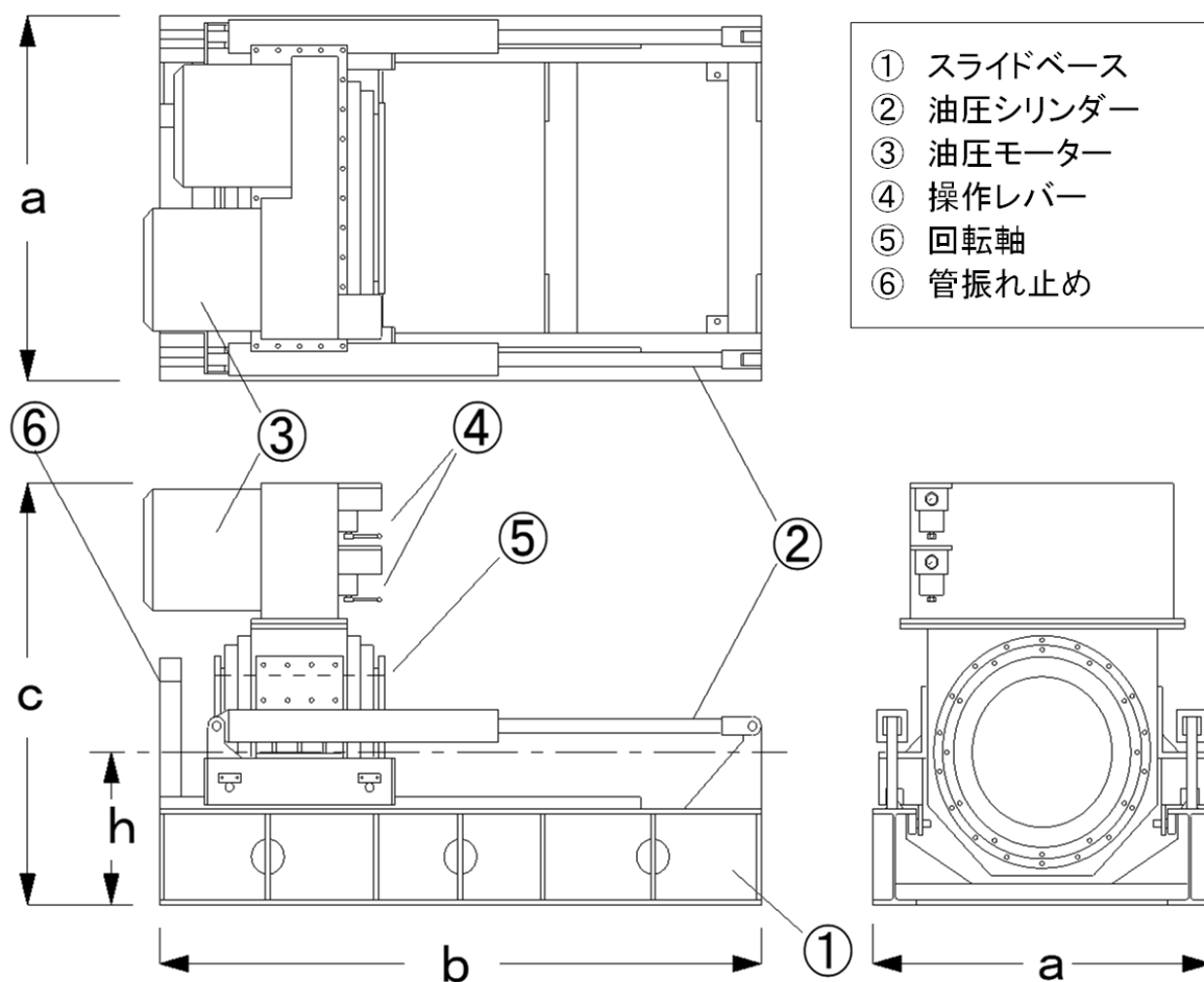
図ー4 ハードロック工法推進機
