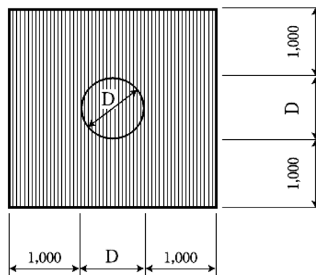
図－7－1 地盤改良断面例
