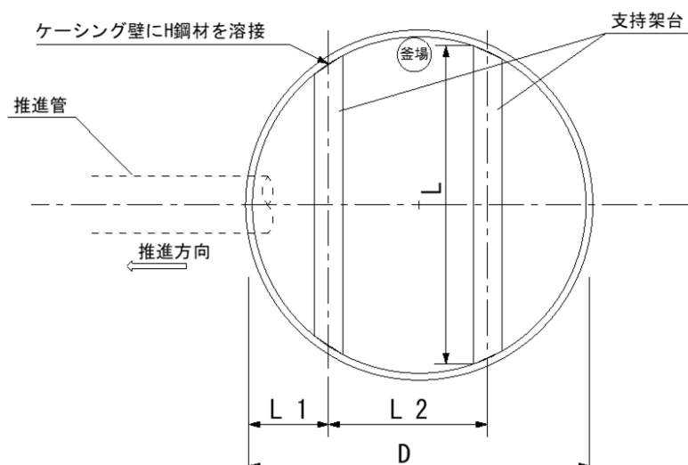
断面図
