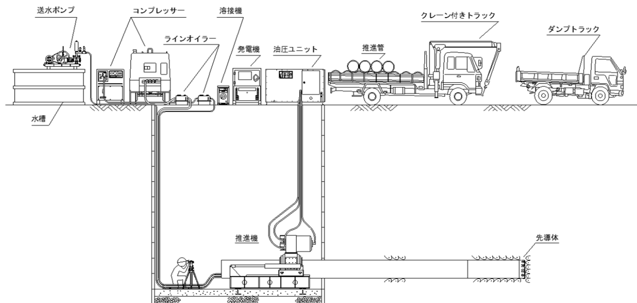
図-1 ハードロック工法施工概要図
